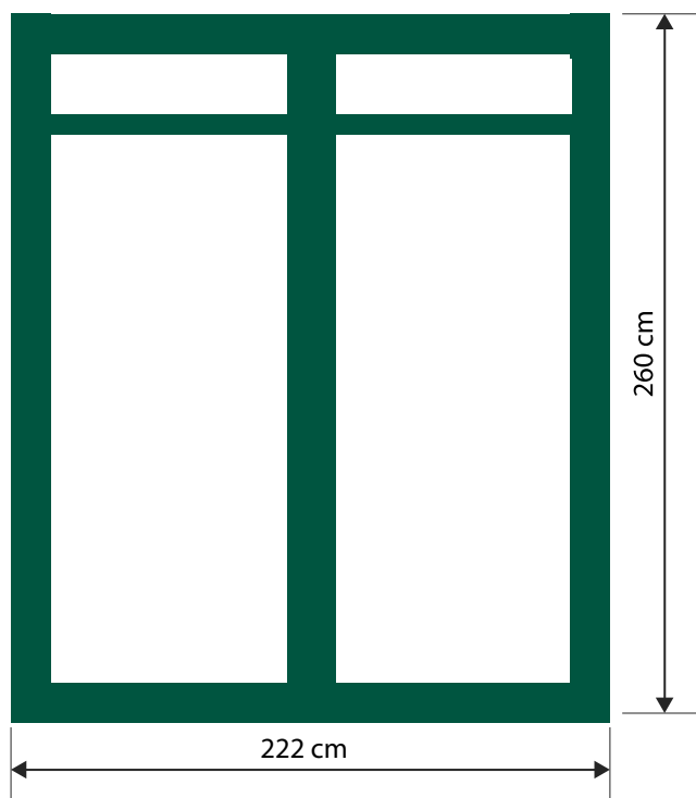
Alzado
